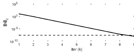
Fig. 3 – Norma 2 de s ( \|s\|_2 ) para cada iteración k
