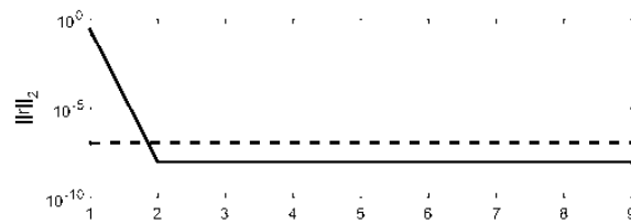
Fig. 2 – Norma 2 de r ( \|r\|_2 ) para cada iteración k
