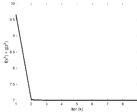
Fig. 1 – f(x) + g(z) para la iteración k
