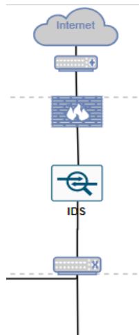
Fig. 2 – Estructura de red basada en sistema de detección de intrusiones a nivel de red, observar que el IDS Snort se coloca después del cortafuego externo.
