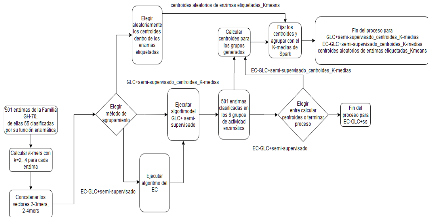
Fig. 2 – Flujo de procesos del agrupamiento de enzimas.
