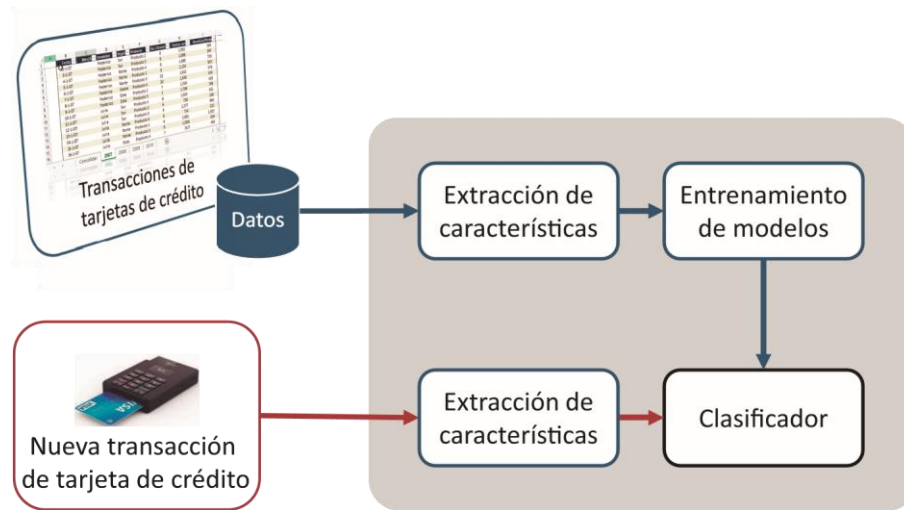
Figura 3. Flujo de un método de detección de anomalía tomando como datos transacciones de tarjetas de créditos.
